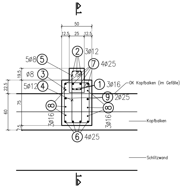
Schnitt 2-2
